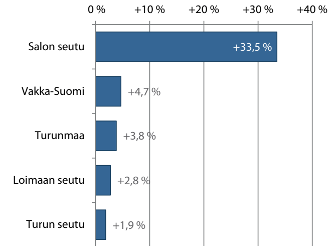
Tilastointitavan muutoksen laskennallinen vaikutus BKT:een vuonna 2011 (%)
